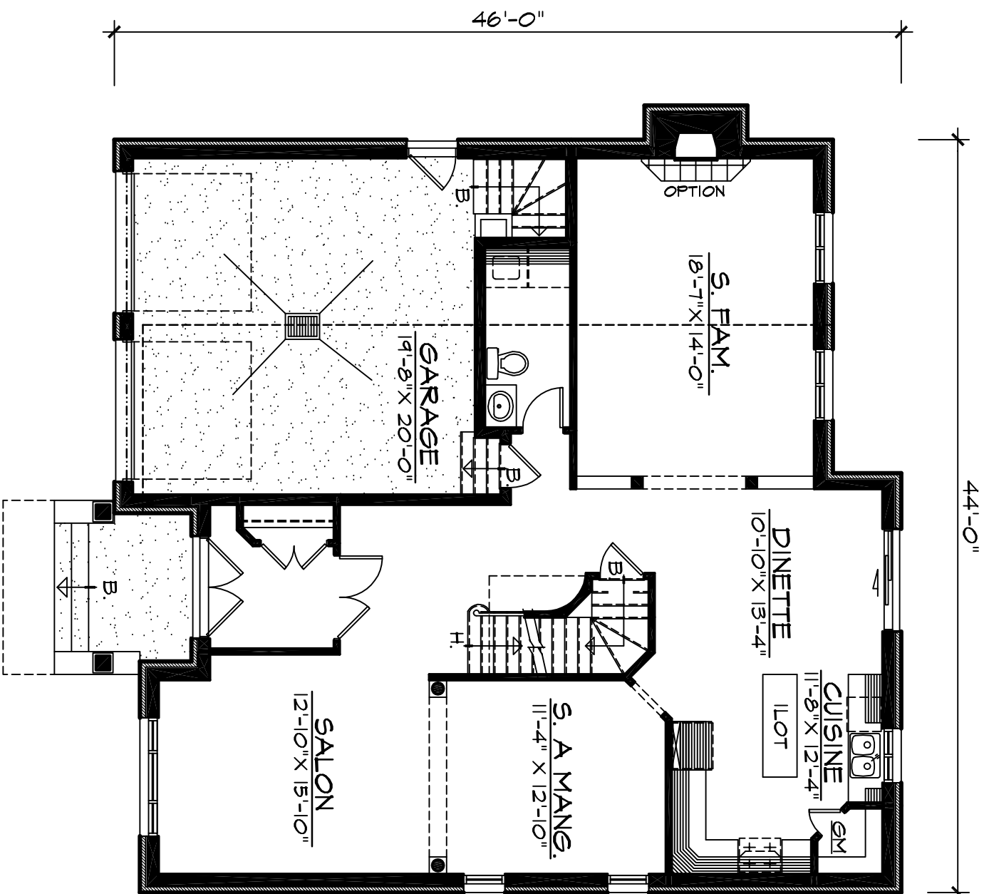
REZ-DE-CHAUSSÉE (1409 pl. car. GARAGE: 478 pl. car.) FOYER EN OPTION.
